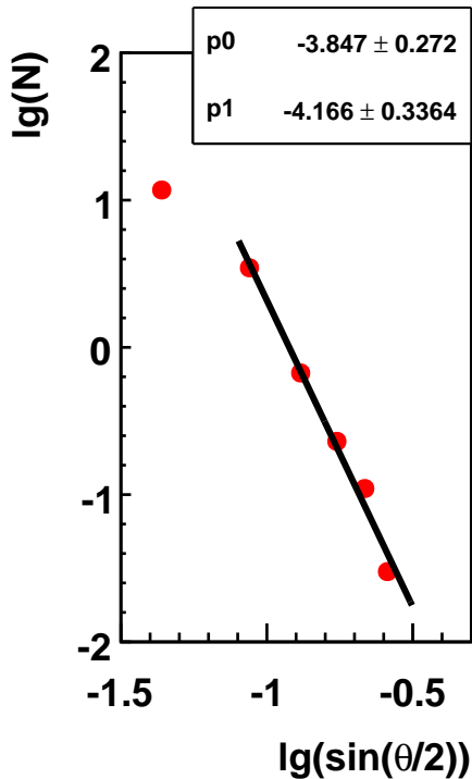
Rutherford Streuung
